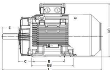
CARCAÇAS 71 A 160
